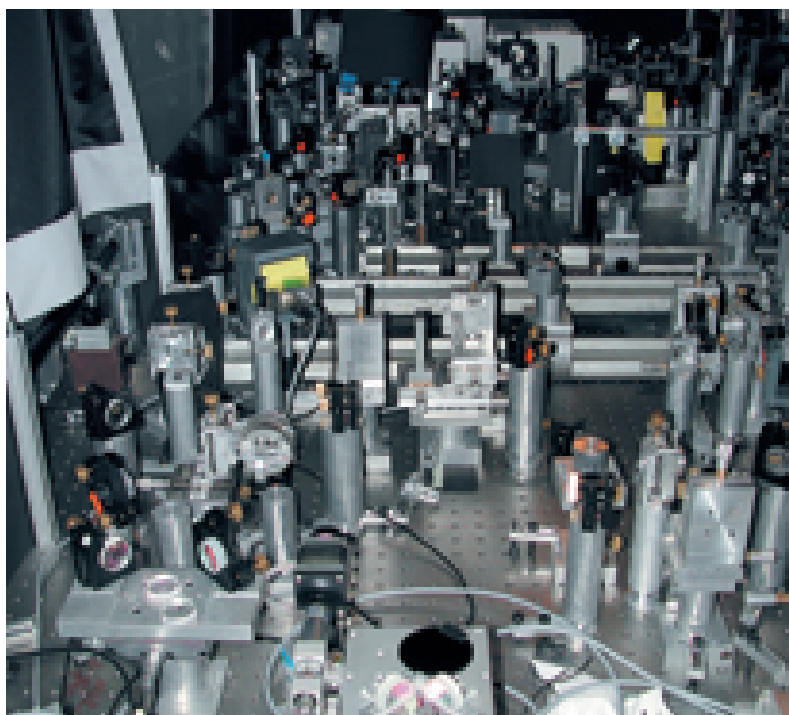
3 Die experimentelle Realisierung eines Kurzzeitlaser-Experimentes im Labor. Links: So genannter Superfluoreszenzring, der bei der Erzeugung farblich abstimmbarer kurzer Lichtimpulse entsteht; rechts: Ausschnitt aus der fs-Laserapparatur.
